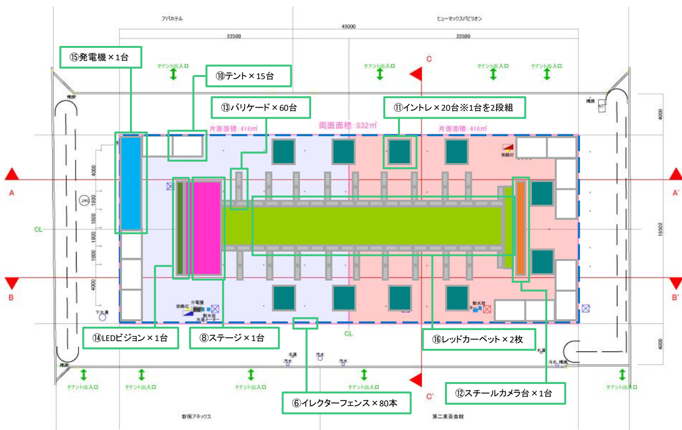
【イントレ(1段組)】
