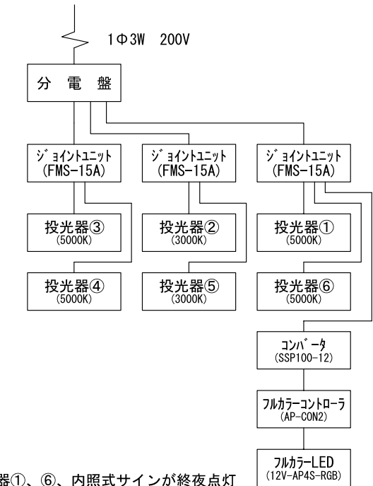
電 気 配 線 図
