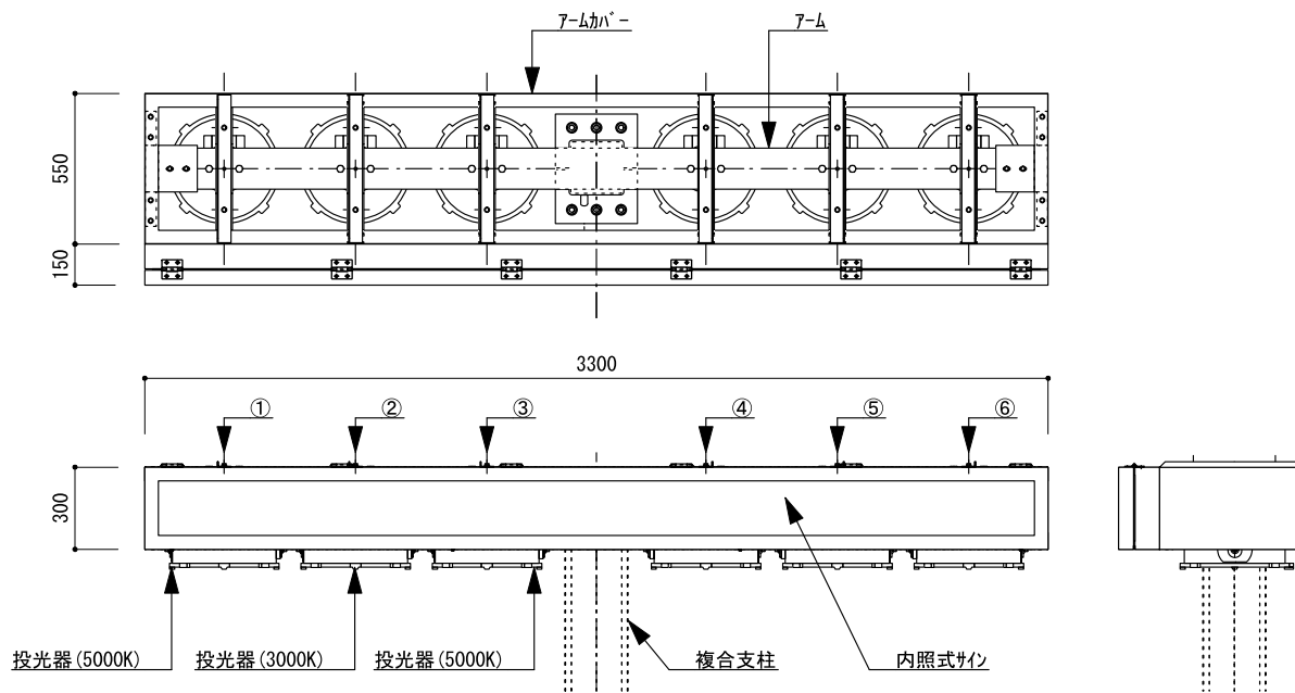
内照式サイン S=1/30
