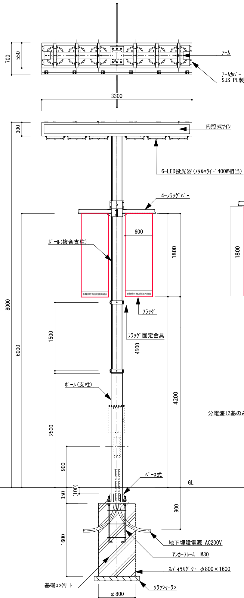
全体図 S=1/50
